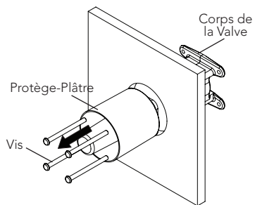
Adaptateurs (2)
