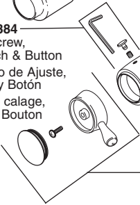
RP51426▲ Temperature Knob, Cover & Screw Perilla de la Temperatura, Cubierta y Tornillo Poignée de Réglae de Température et Vis
