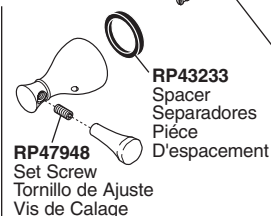
H740▲ Handle Kit Juego de herrajes de la Manija Manette en kit
