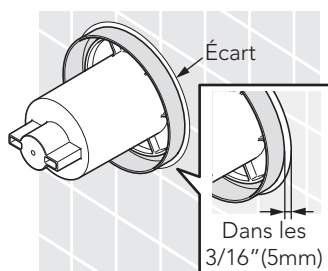
Calfeutre adhésif
