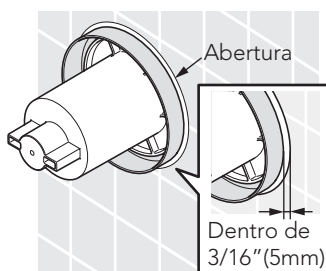
Calafetar adesivo
