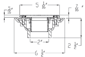
Section A-A LW 5
