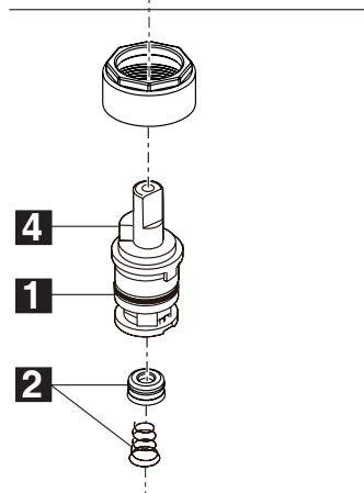
RP100687 Stem Unit Assembly, Seat & Spring, Bonnet Nut Ensamble de la Unidad del Vástago, Asiento y Resorte, Bonete Obturbateur, siège et ressort, écrou à chapeau
