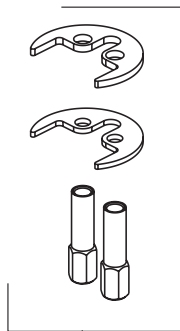
RP33126 Mounting Hardware Pièces de montage Herraje de instalación
