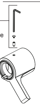
RP75442▲ Handle, Set Screw, Button & Wrench Manija, Tornillo de Ajuste, Botón y Llave Poignée, Vis de calage, Bouton et Clé
