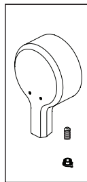
RP91910 ▲ Temperature Handle, Set Screw & Button Manija de la temperatura, tornillo de ajuste y botón Manette de température, vis de calage et bouton
