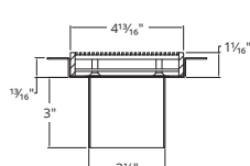
Section A-A FFAS 125
